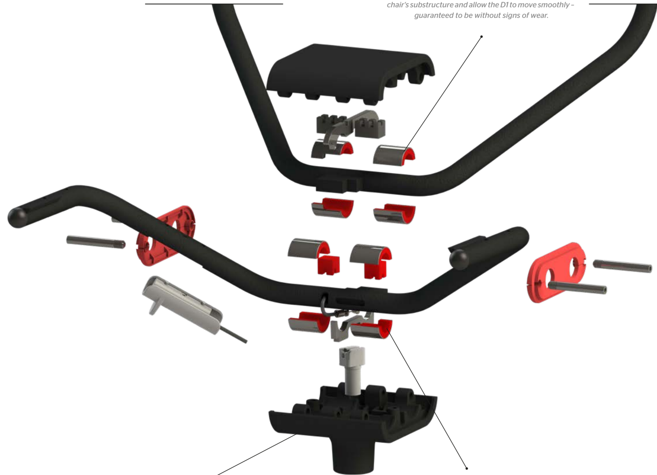
GEHÄUSE CASING
